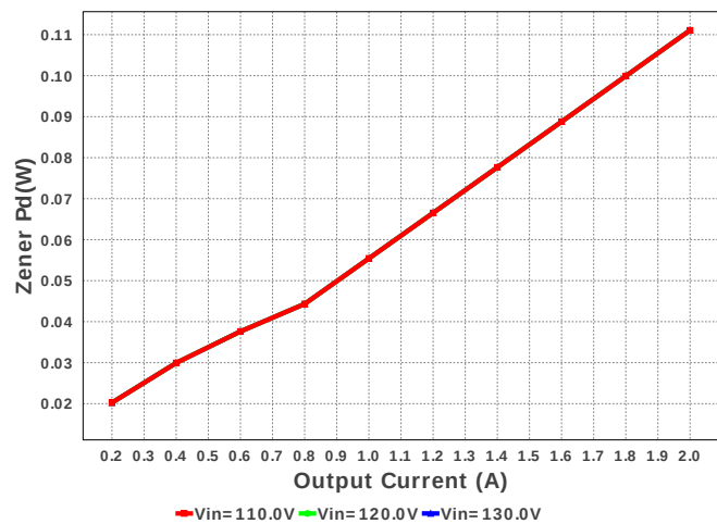
Zener Pd
