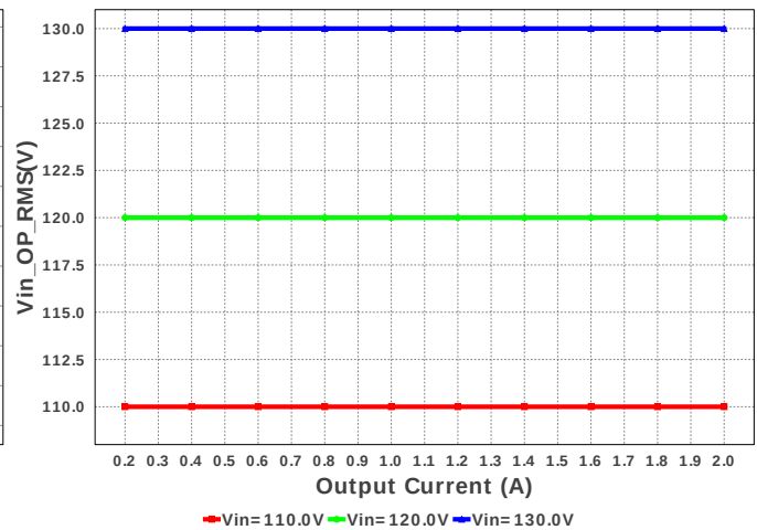
Vin_OP_RMS
