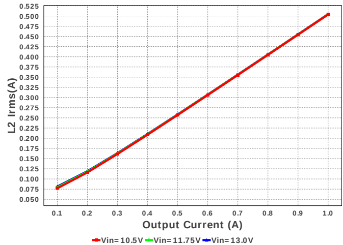
L2 Irms
