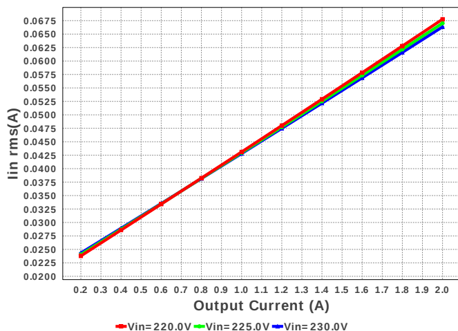
Iin rms
