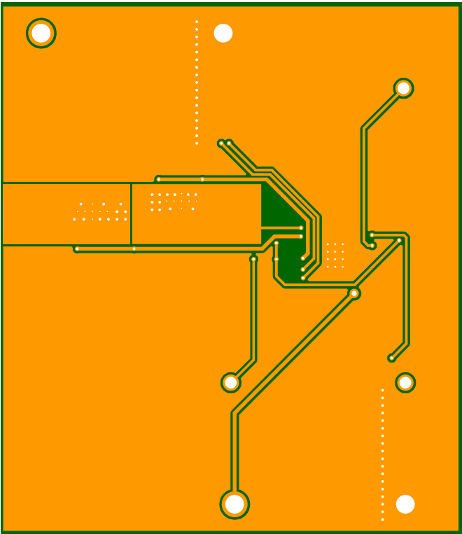
Bottom Layer
