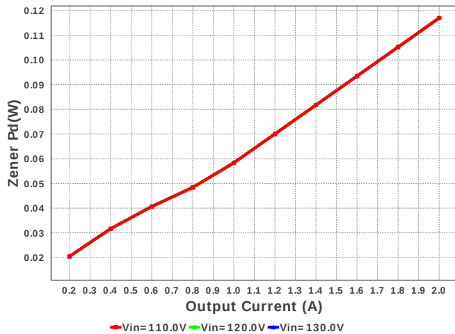
Zener Pd
